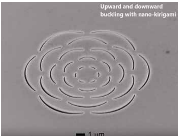
集束イオンビームを金属箔に照射して作成した、ナノスケールのパターン。 自然界ではありえない振る舞いを電磁波にさせることが可能になる。Image by MIT
